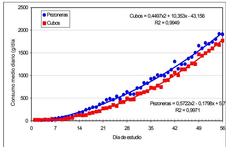
Figura 3. Ajuste por mínimos cuadrados del consumo diario de pienso de arranque (en base a materia seca).
